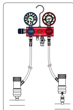
ゲージマニホールド 接続時
